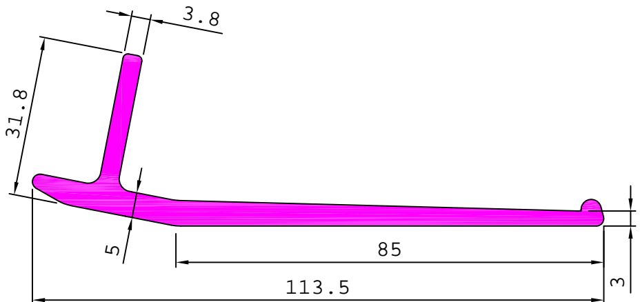
18637 1.584 kg/m
