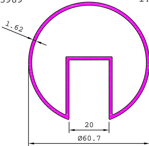
S3989 1.069 kg/m
