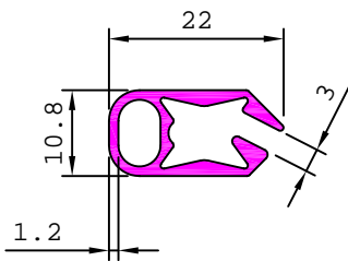
S4083 0.228 kg/m
