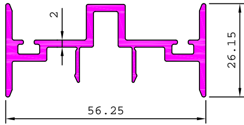
S3989 1.069 kg/m
